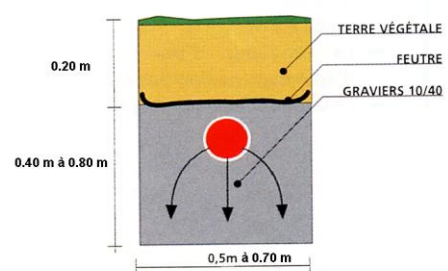
COUPE D'UNE TRANCÉE
